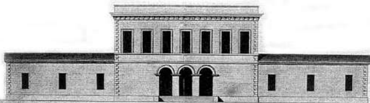
ÉLEVATION ET COUPE de l'Hôtel-de-Ville de Napoléon (Vendée.)
